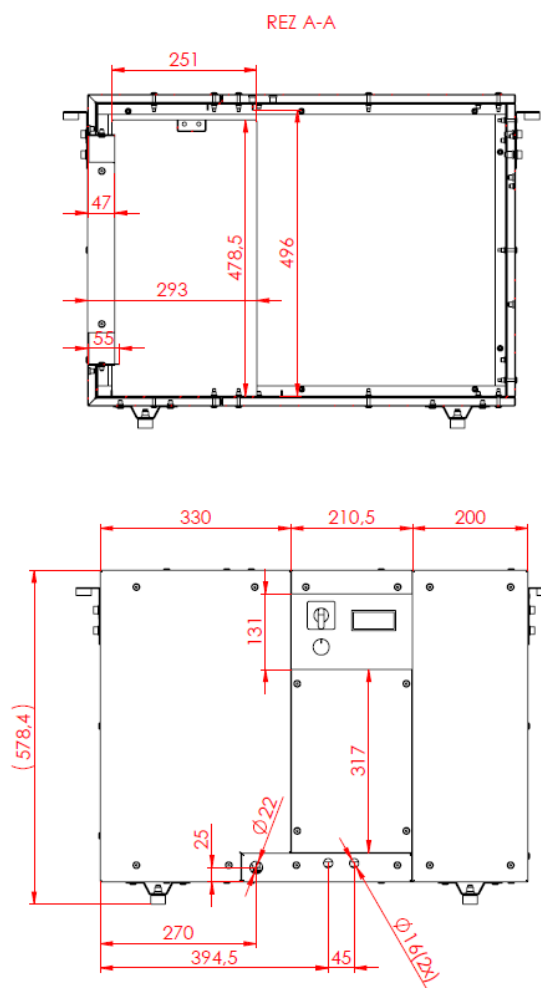
Boční pohled
